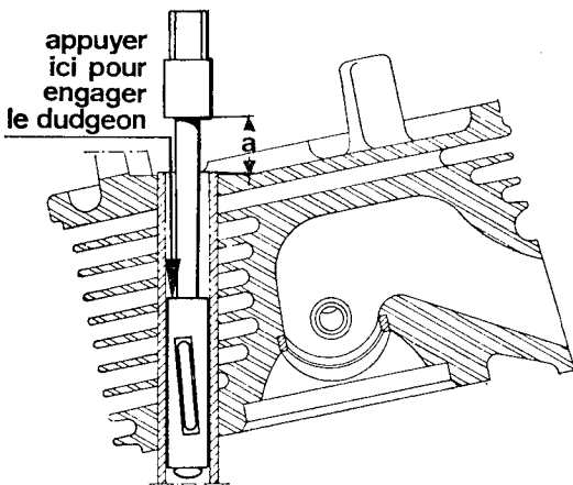
Dudgeonnage de la partie inférieure d'un tube de tige de culbuteur (outil 1605-T)
